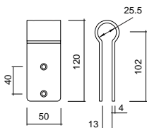
Suporte Superior
