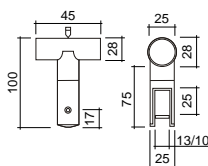
Suporte Superior
