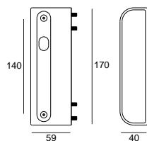
Fechadura Testa
