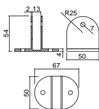
Suporte Lateral
