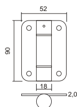
Dobradiça com Mola
