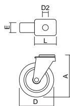
Roda Giratória Poliamida com Furo
