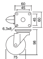
Roda sem Travão
