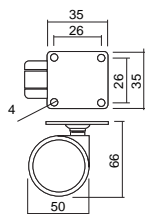
Roda Giratória com Base sem Travão
