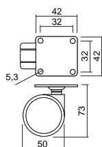
Roda com Travão com Base
