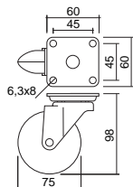
Roda com Travão
