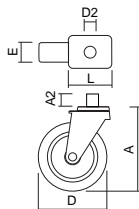
Roda Giratória Poliamida com Parafuso
