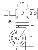
Roda Giratória Poliamida com Base
