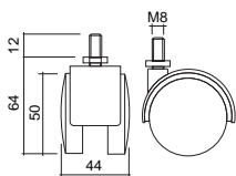
Roda Cadeira com Perno sem Travão
