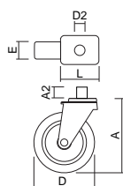
Roda Giratória Poliamida com Furo
