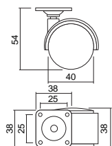
Roda Cadeira com Base sem Travão
