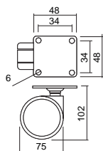
Roda Giratória com Base sem Travão
