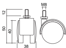
Roda Cadeira com Perno com Travão
