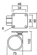
Roda Giratória com Base com travão
