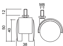
Roda Cadeira com Perno sem Travão
