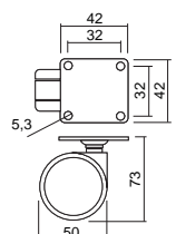
Roda sem Travão com Base
