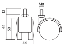
Roda Cadeira com Base com travão
