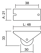
Roda Fixa com Base sem Travão
