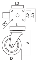
Roda sem Travão
