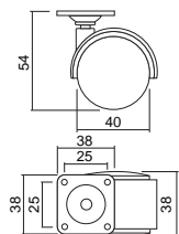
Roda Cadeira com Base com travão
